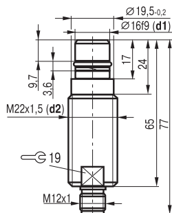
Габаритный чертёж
